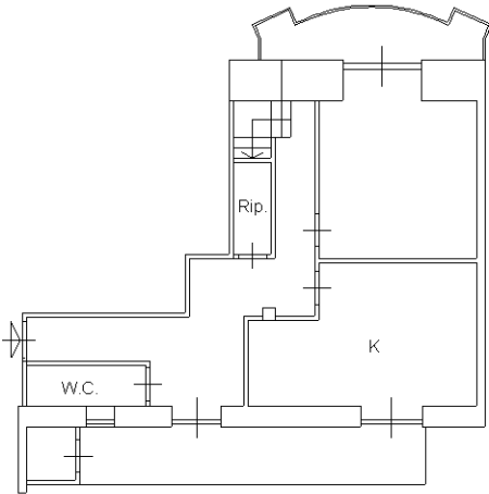
PIANO SECONDO
